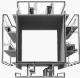
SQUARE POLE 54 SP ( 4 WAY POLE )
