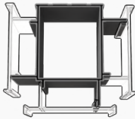
TEE POLE 45 TP ( 3 WAY POLE )
